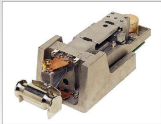
SHS weegsensor met auto kalibratiegewicht
